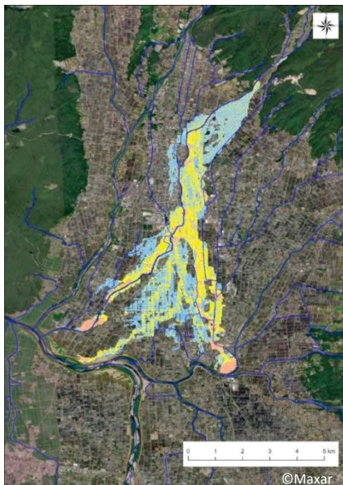
■ 田んぼダム実施による浸水深・浸水面積の軽減イメージ（阿賀野川水系田付川流域）
